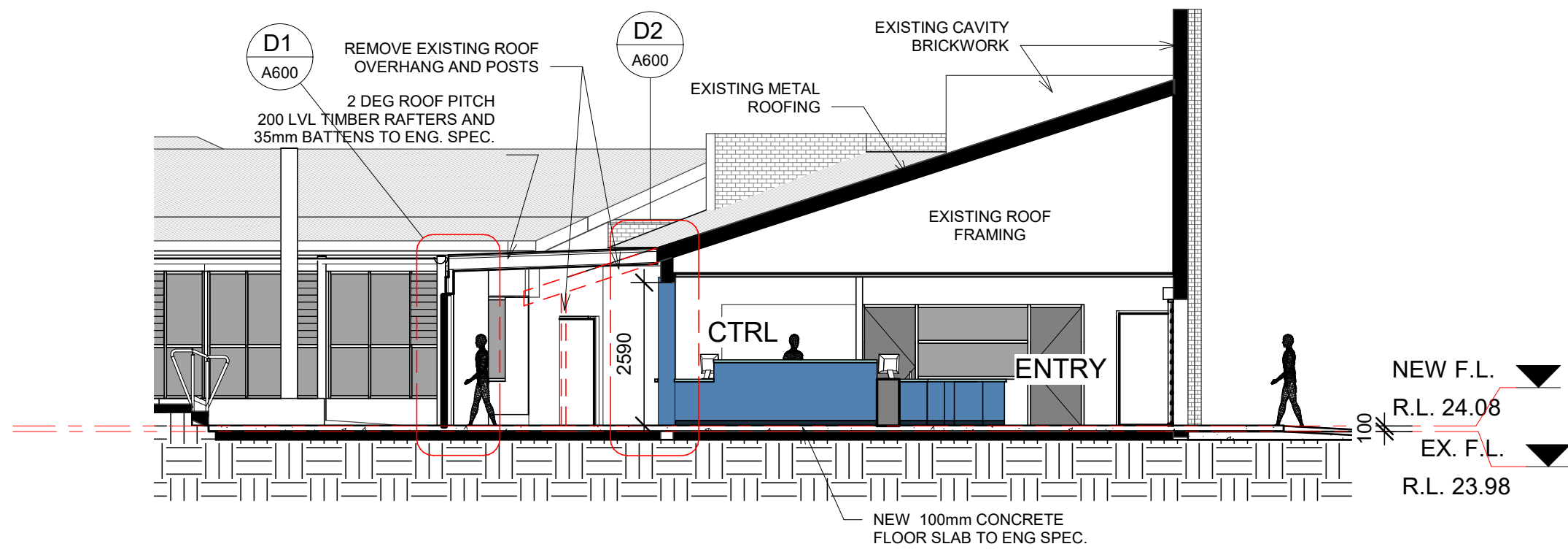
SECTION B 1 : 100
