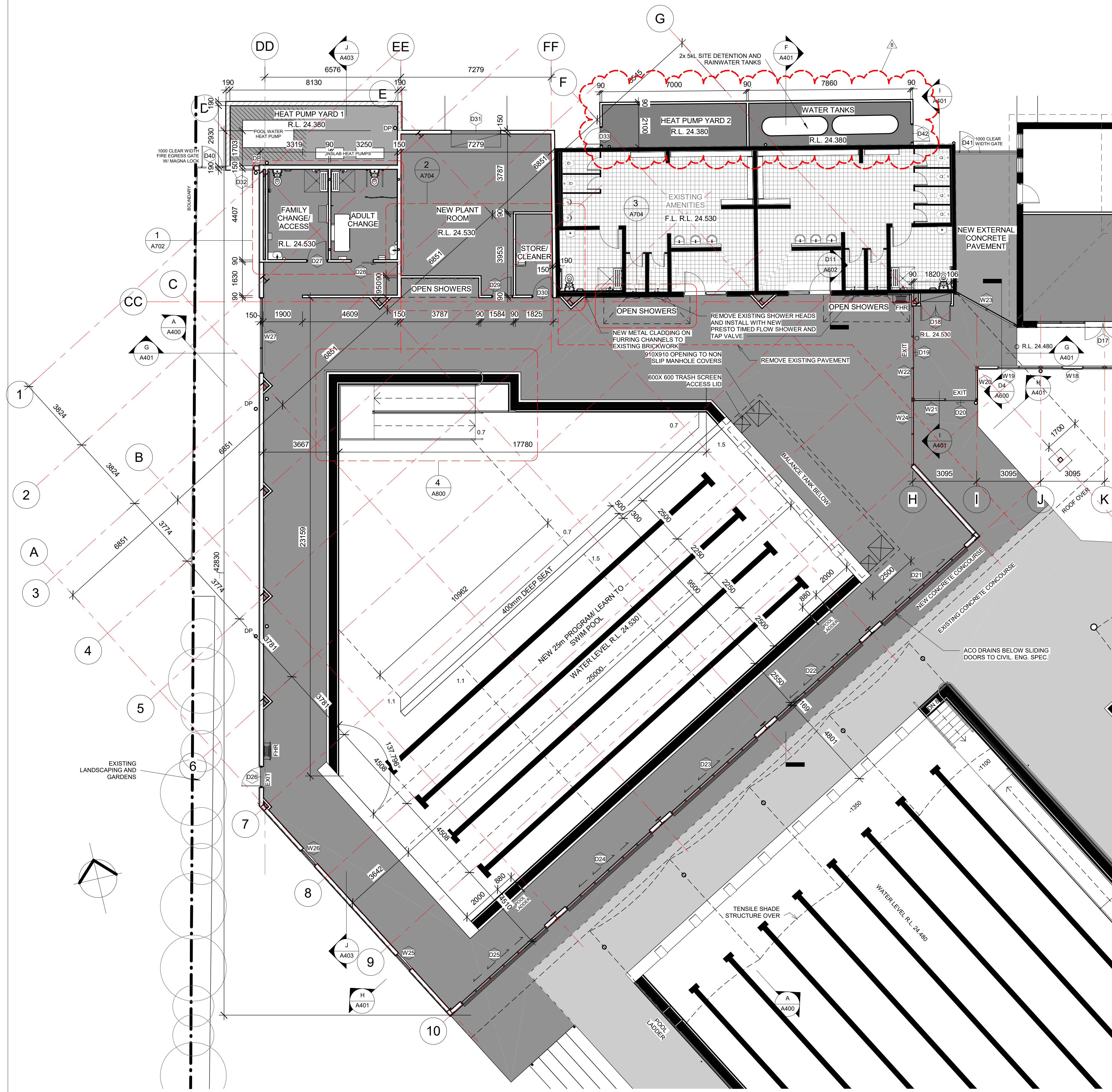
FLOOR PLAN 3 1 : 100
