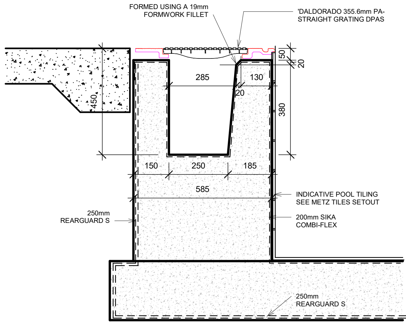
GUTTER DETAIL 1 : 10
