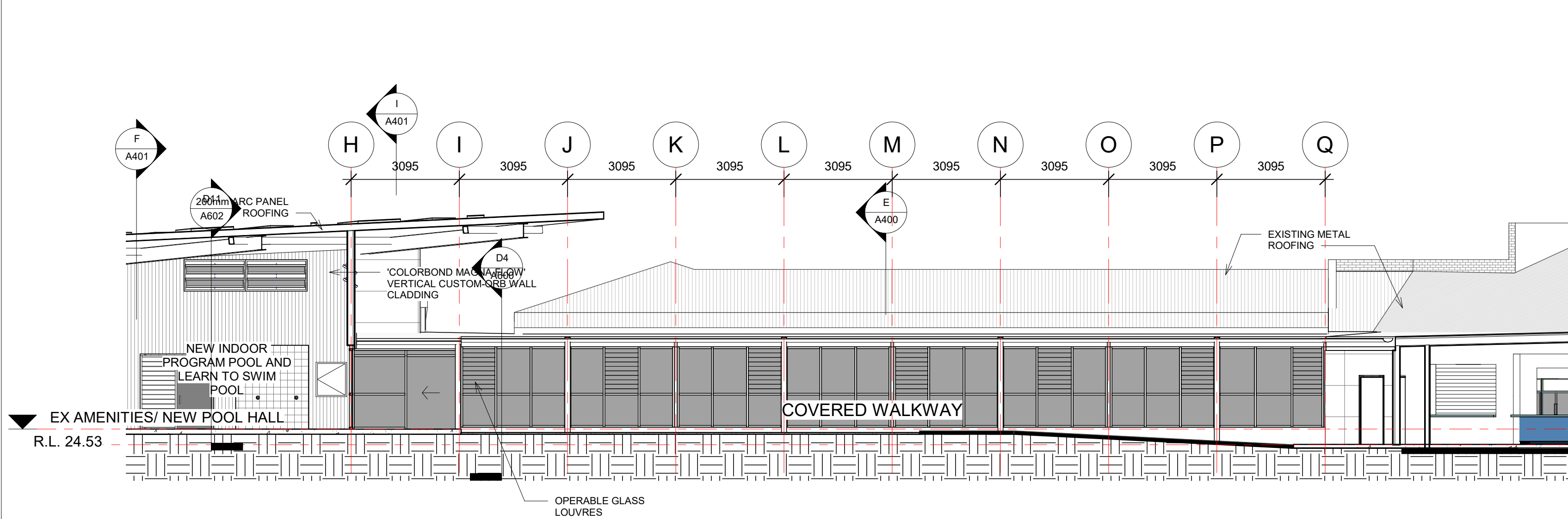
SECTION D 1 : 100
