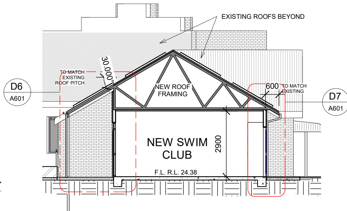
SECTION C 1 : 100
