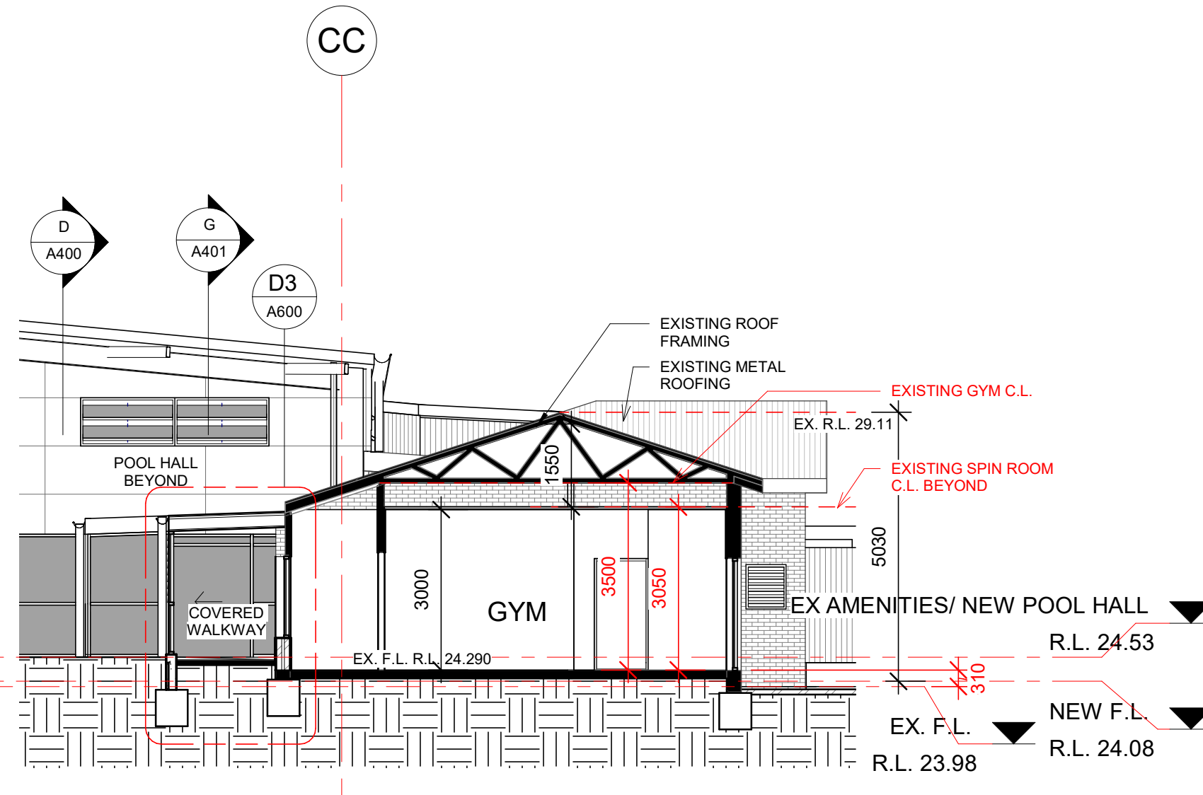
SECTION E 1 : 100
