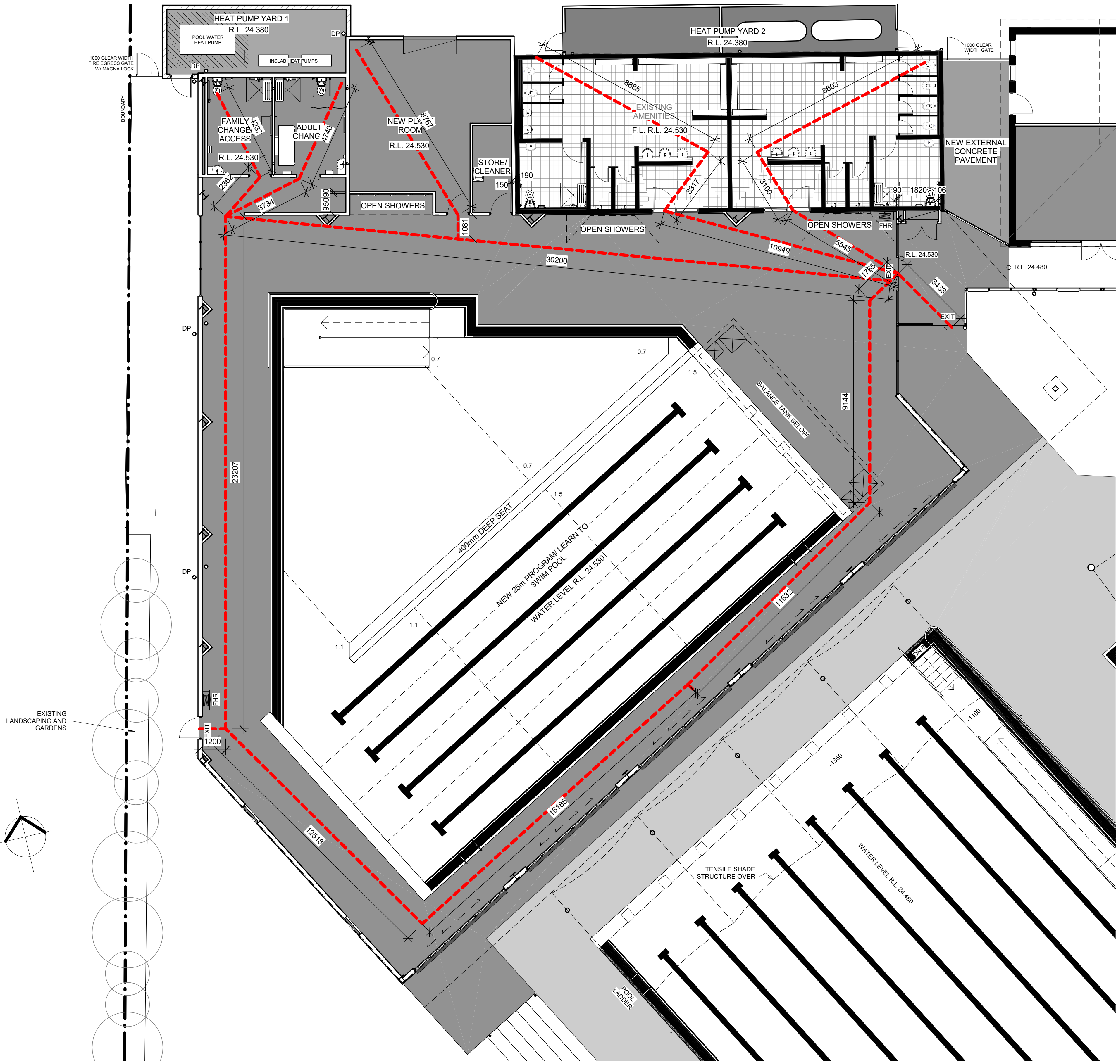
EGRESS PLAN 3 1 : 100
